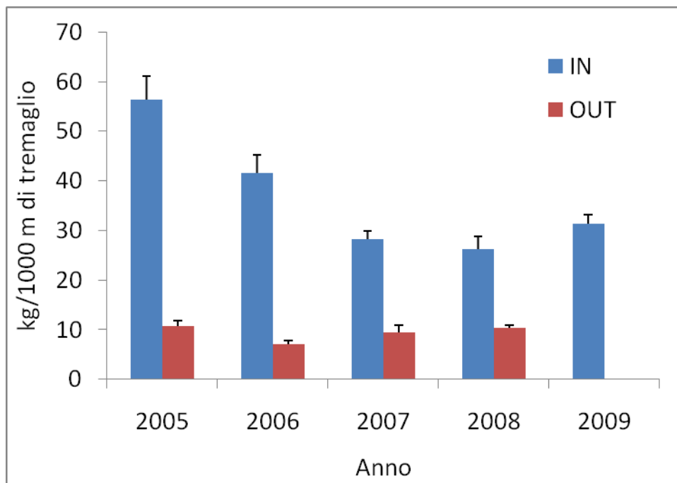
Figura 3.2.2. Rendimenti di pesca medi ( \pm SE) annuali (2005-2009) all'interno (zona C) ed all'esterno dell'AMP di Torre Guaceto.
