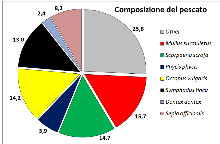
Figura 3.2.1. Composizione percentuale delle catture (peso fresco) effettuate in zona C dell'AMP di Torre Guaceto.
