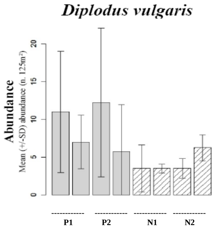
Figura 3.1.3. Abbondanza di Diplodus vulgaris nelle due località protette (P1 e P2) dell'AMP di Torre Guaceto e non protette (N1 e N2).
