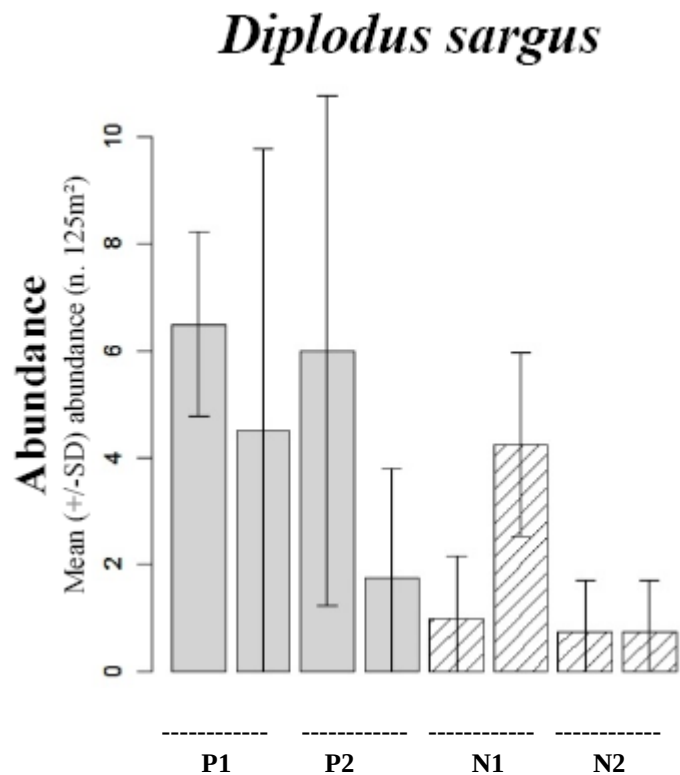
Figura 3.1.1. Abbondanza di Diplodus sargus nelle due località protette (P1 e P2) dell'AMP di Torre Guaceto e non protette (N1 e N2).
