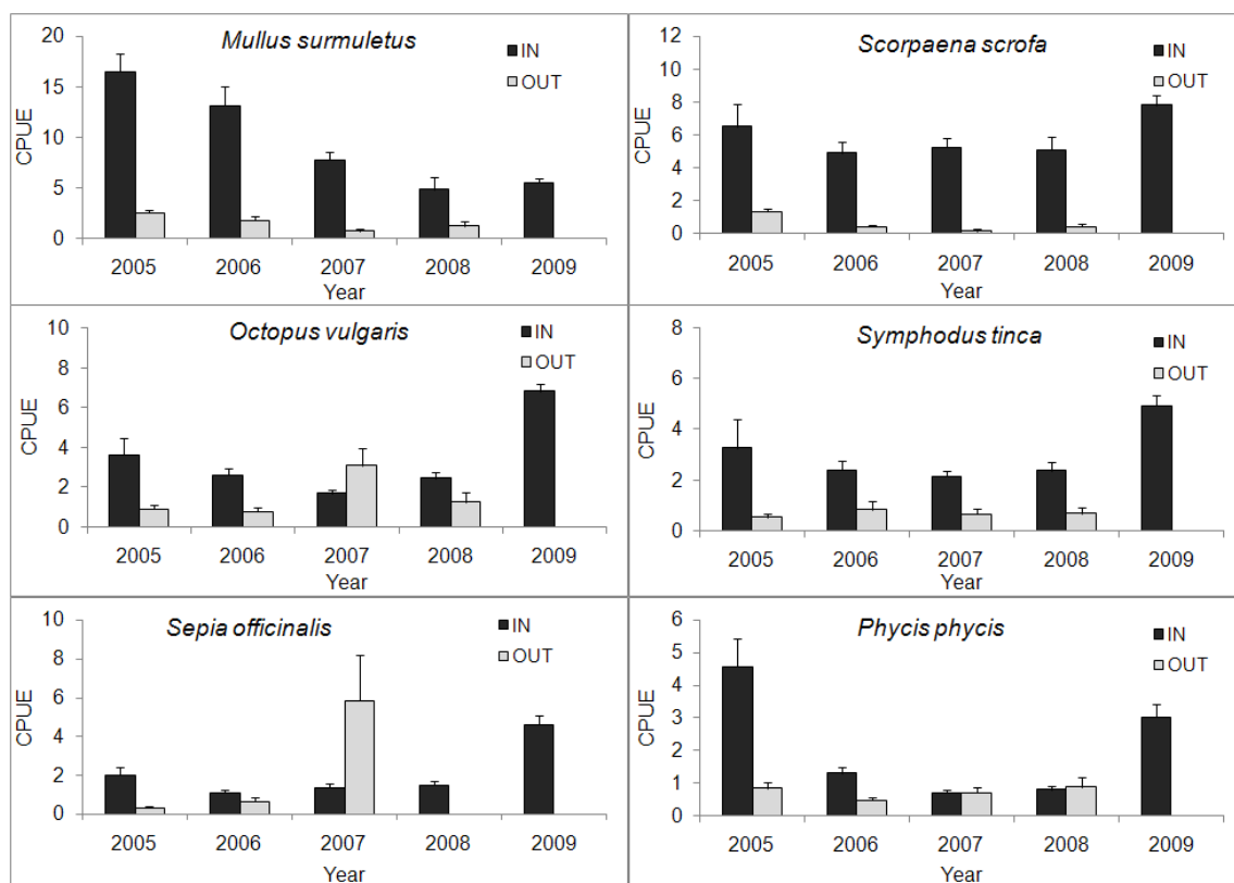
Figura 3.2.3. Rendimenti di pesca (kg/1000 m di rete; media \pm SE) di 6 specie bersaglio presso la zona C dell'AMP di Torre Guaceto dal 2005 al 2009.
