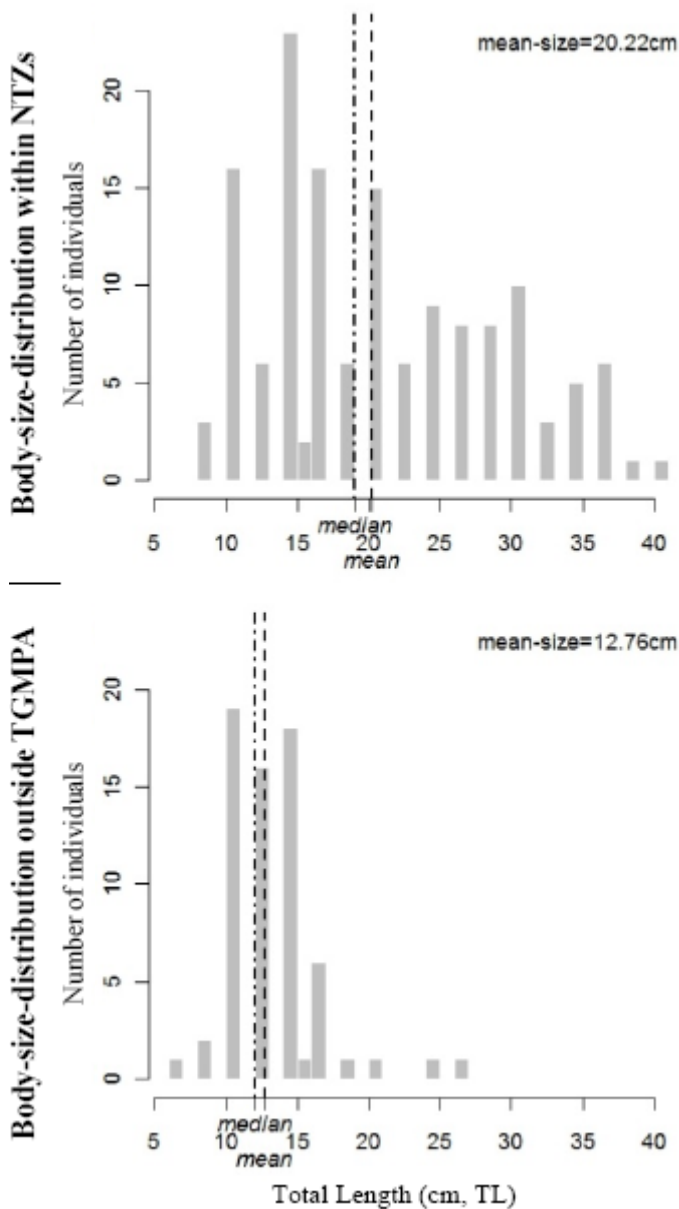
Figura 3.1.4. Distribuzioni di taglia (lunghezza totale, cm) di Diplodus vulgaris nelle località protette (NTZs: no-take zones) dell'AMP di Torre Guaceto e non protette al di fuori dell'AMP (outside TGMPA).
