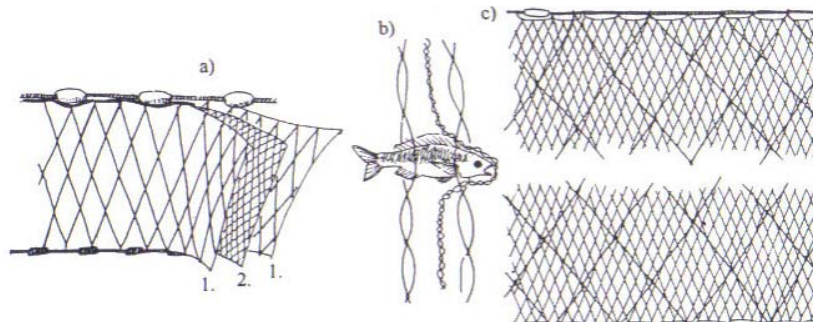
Figura 2.2.1. Struttura generale e dinamica di cattura del pesca del tremaglio.
